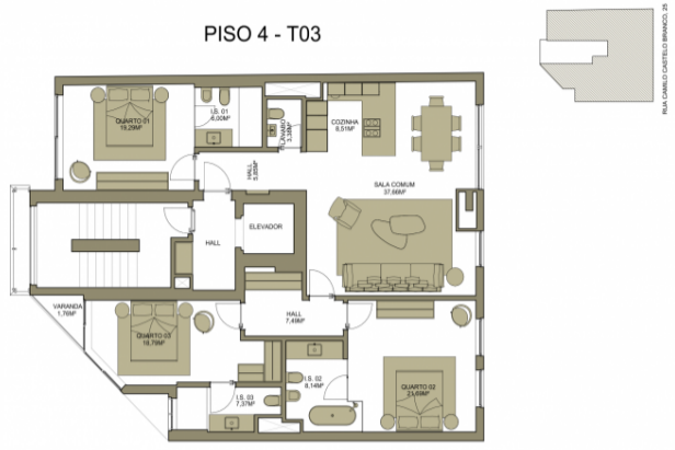
PISO 4 - T03 Escala: 1/100
